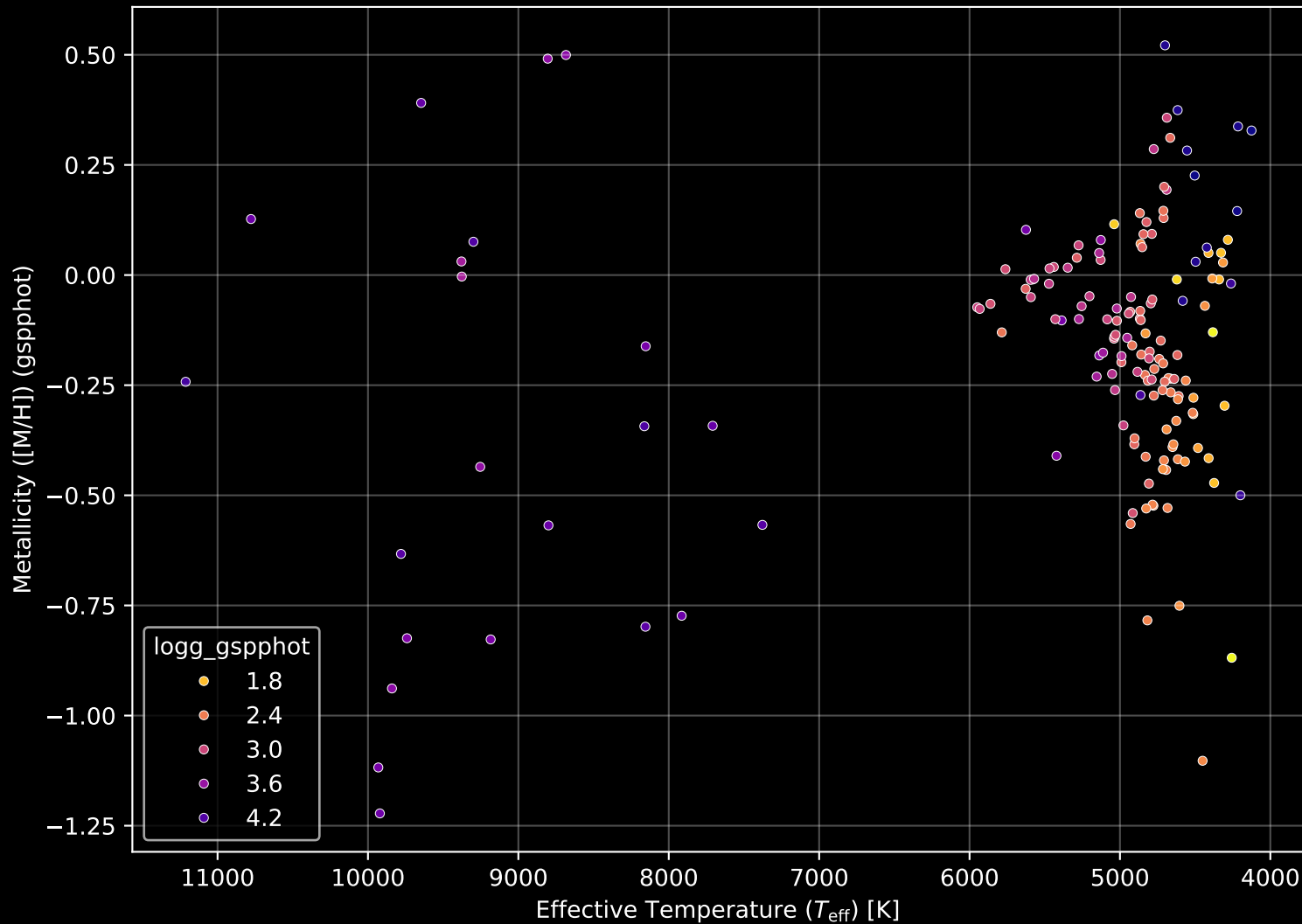
APOGEE DR17 Field: [235+12] Stellar Population Parameters (n= 161)
